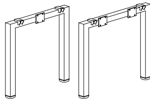
N LEG (END) MUN1800(E) L1790 x H725 MUN1500(E) L1490 x H725 MUN1200(E) L1190 x H725 MUN1050(E) L1040 x H725 MUN 900(E) L890 x H725 MUN 750(E) L740 x H725 MUN 600(E) L590 x H725
